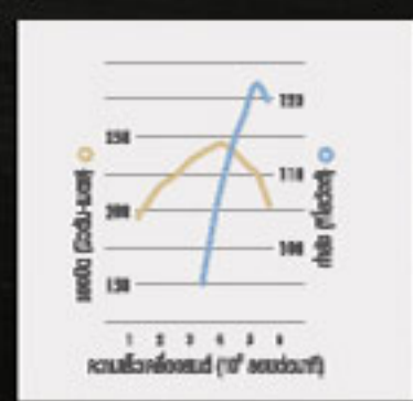
เครื่องยนต์เบนซิน 2.7 ลิตร Dual VVT-i* (เกียร์ธรรมดา 5 สปีด)
