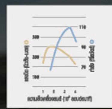
เครื่องยนต์ดีเซล 2.4 ลิตร (เกียร์ธรรมดา 6 สปีด / เกียร์อัตโนมัติ 6 สปีด)
